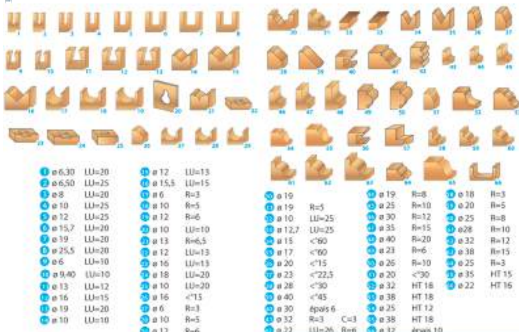
DEF.428.14 COFFRET DE 12+2 MÈCHES DE DÉFONCEUSE
