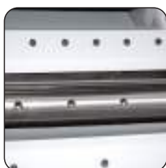
Arbre de dégauchissage de Ø70mm avec 3 fers 310x25x3.
