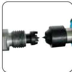
Alignement des pointes CM2 et broche d'entraînement fileté M33 x 3,5 mm
